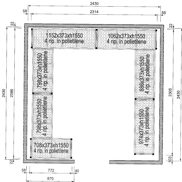
Boven aanzicht
